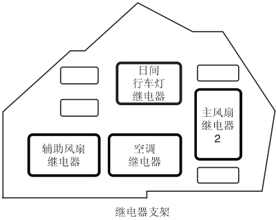
继电器支架
