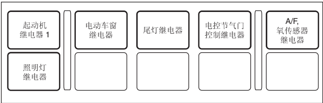
继电器支架（左驾车型）
