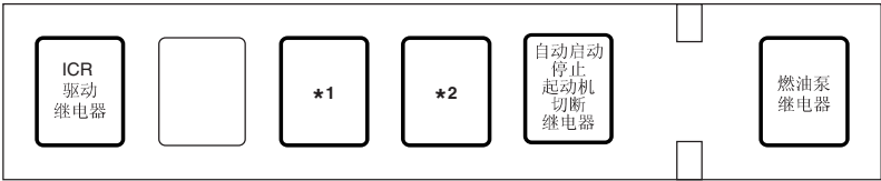
继电器支架 (自动启动停止)
